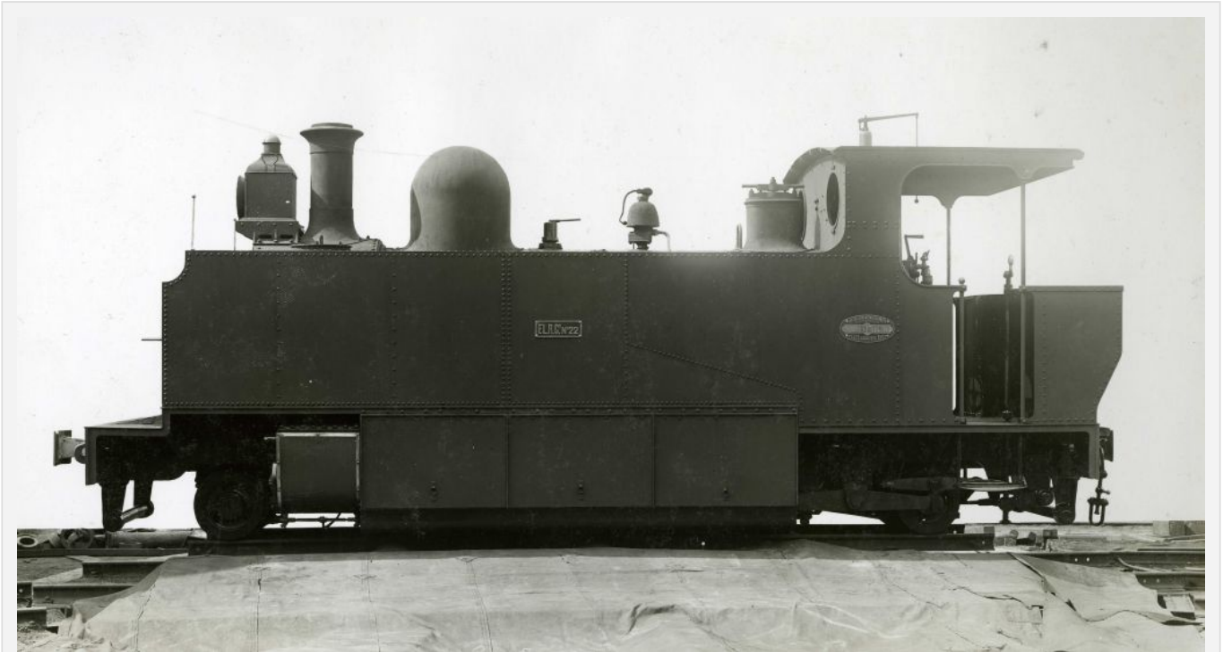
Tubize 1521 de 1907 pour le FLR (n° 22). Photographie d'usine, coll. Musée 'de la Porte' à Tubize.
