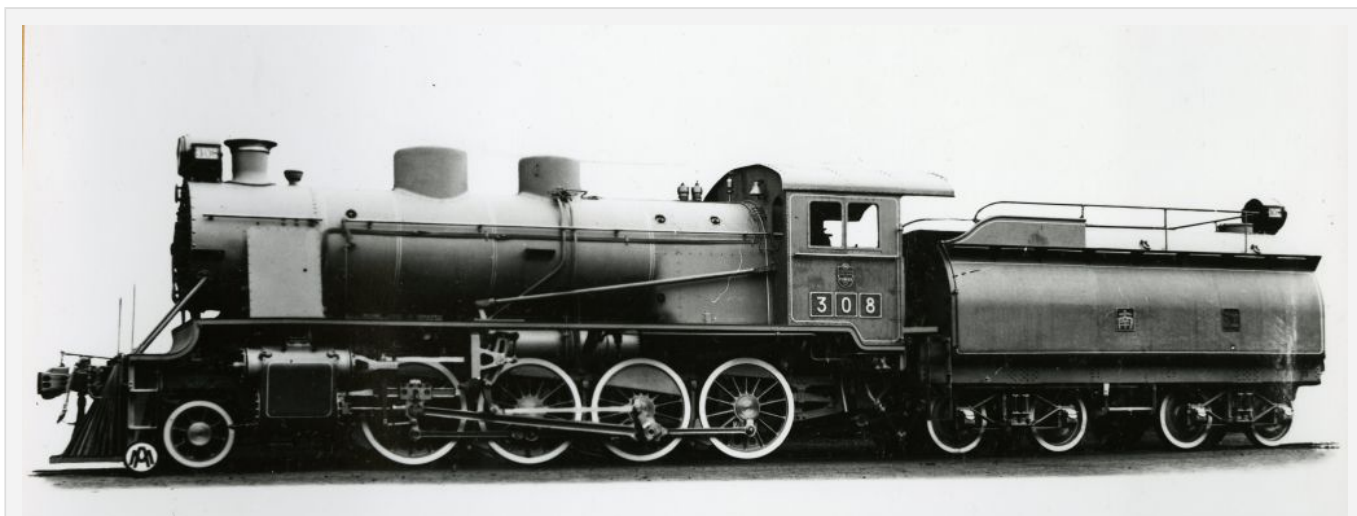
Tubize 2174 de 1934 pour le KiangNan (n° 308). Photographie d'usine, coll. Musée 'de la Porte' à Tubize. Série 2167-2176, 1934, voie 1.435, 1Dh2 ou 2-8-0, KiangNan 301-310.
