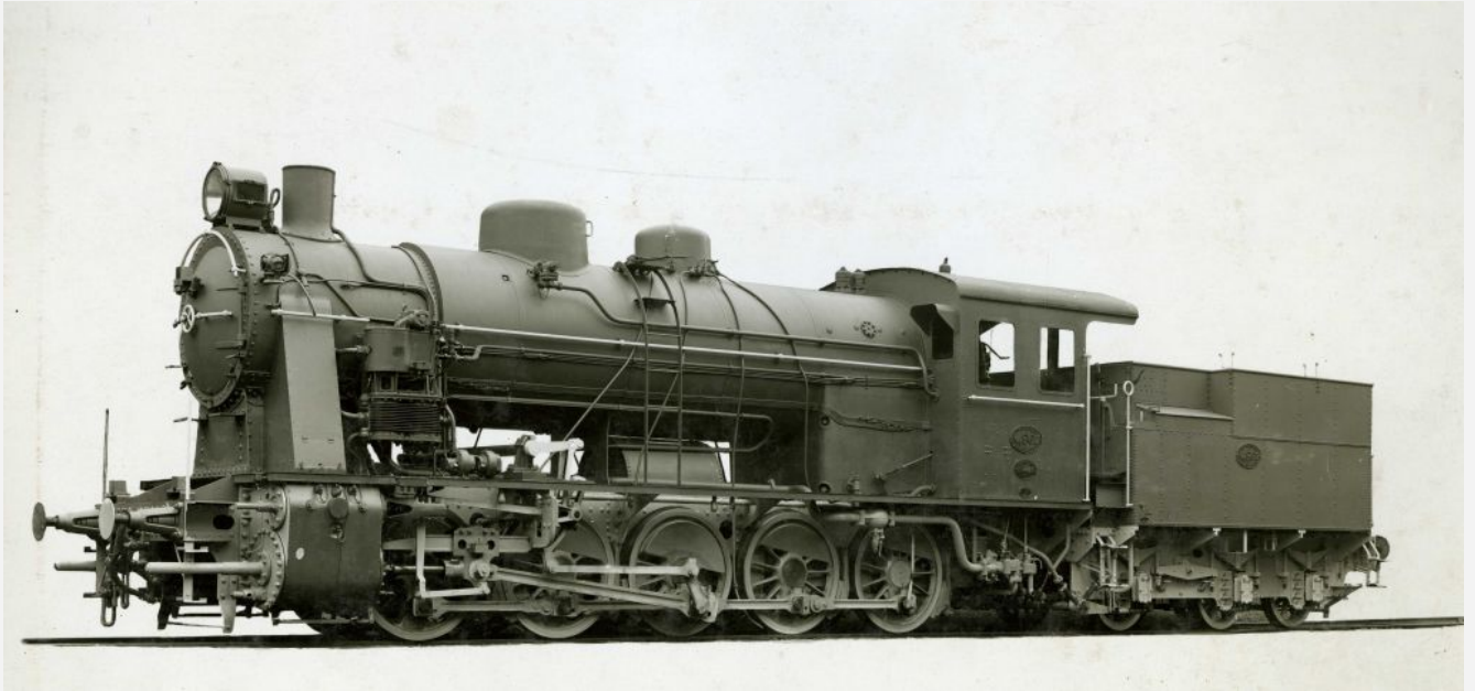
Tubize 2059 de 1927 pour le CEH (n° 867). Photographie d'usine, coll. Musée 'de la Porte' à Tubize. Série 2053-2059, 1927, voie 1.435, Eh2 ou 0-10-0, CEH 861-867.
