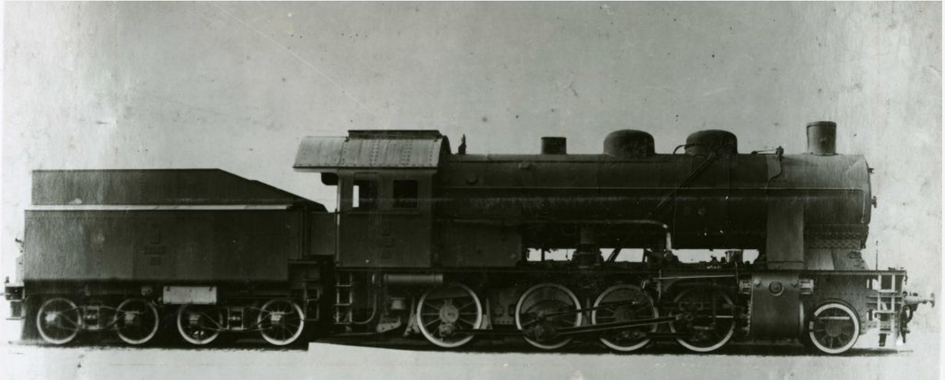
Tubize 1939-1958 de 1924 pour le PKP (n° 21.55-21.74). Photographie d'usine, coll. Musée 'de la Porte' à Tubize. Série 1939-1958, 1924, voie 1.435, 1Dh2 ou 2-8-0, PKP 21.55-21.74.
