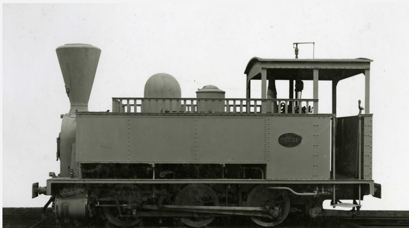
Tubize 1807 DE 1913 pour Bienhoa TONKIN. Photographie d'usine, coll. Musée 'de la Porte' à Tubize. Série 1807, 1913, voie 1.000, Ct ou 0-6-0T.
