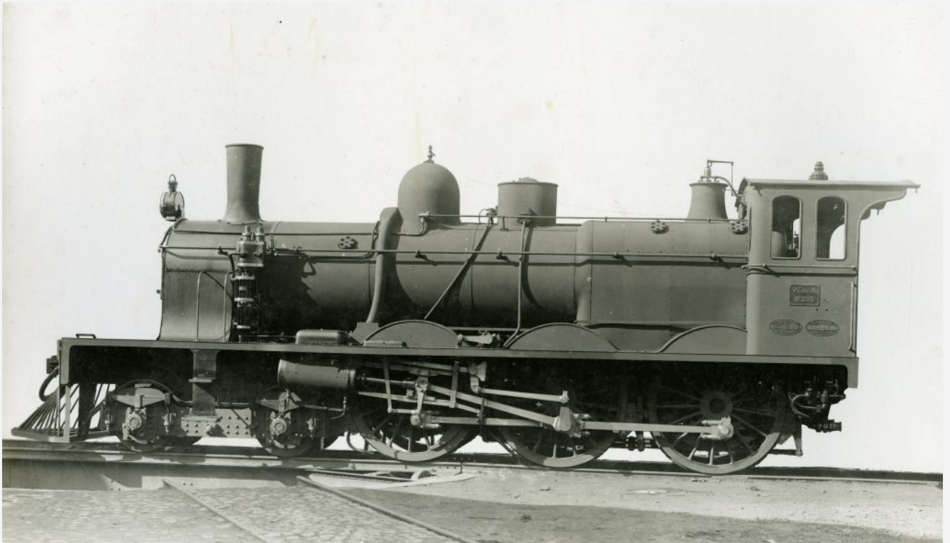
Tubize 1496 de 1906 pour le Pékin - Hankow (n° 230). Photographie d'usine, coll. Musée 'de la Porte' à Tubize.
