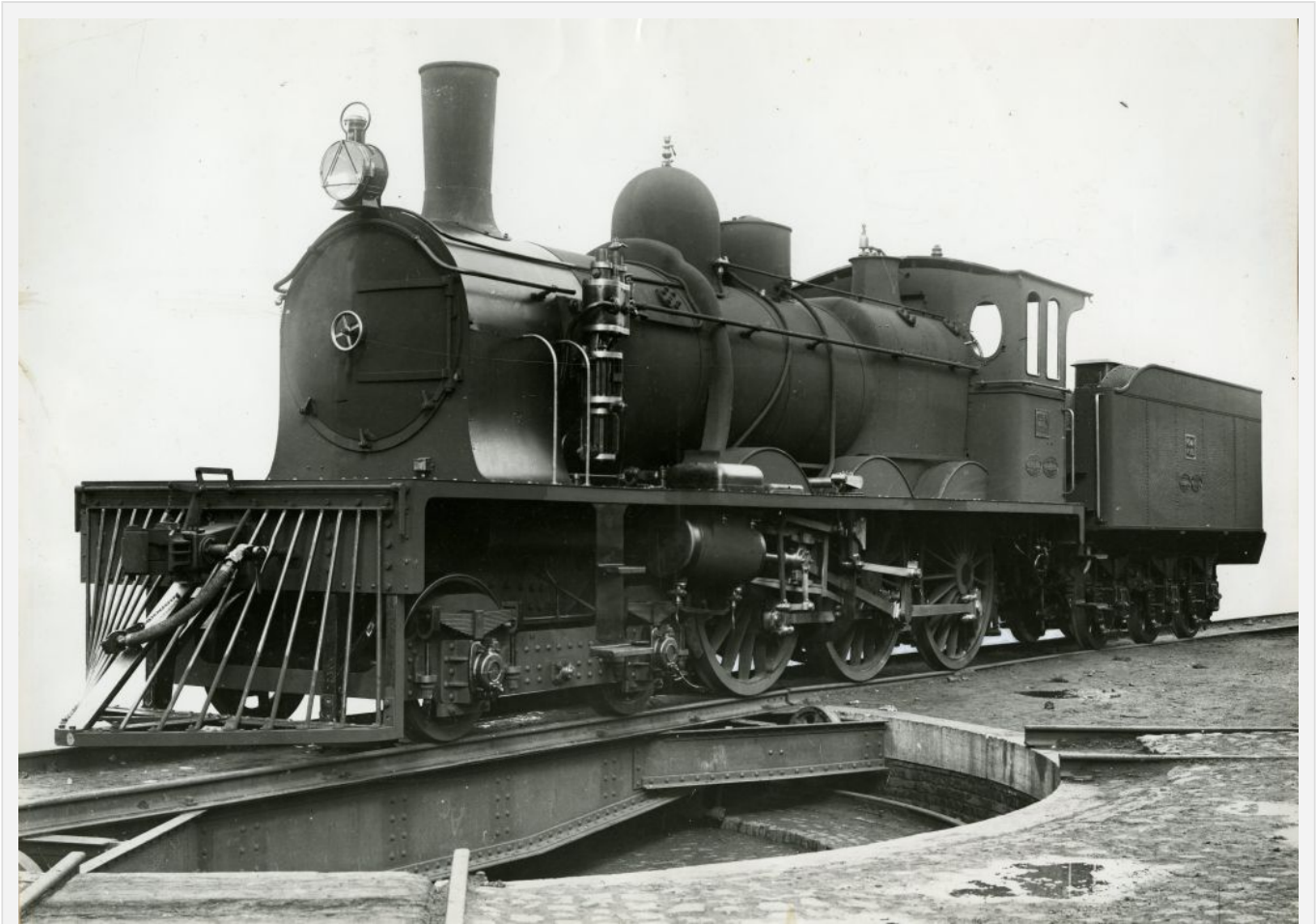
Tubize 1496 de 1906 pour le Pékin - Hankow (n° 230). Photographie d'usine, coll. Musée 'de la Porte' à Tubize.
