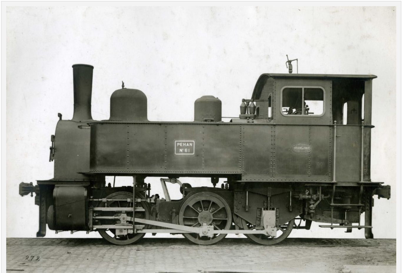
Tubize 1236 de 1900 pour le Pékin-Hankow (n° 61). Photographie d'usine, coll. Musée 'de la Porte' à Tubize
