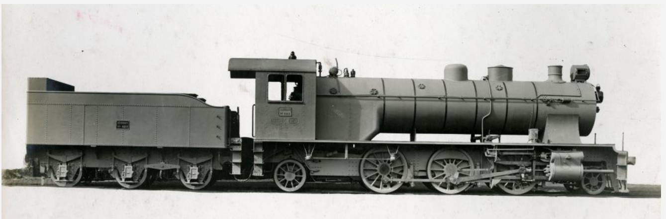
Tubize 1819 de 1921 pour le Peking-Hankow, Kian Han Railway (n° 622). Photographie d'usine, coll. Musée 'de la Porte' à Tubize. Série 1818-1827, 1921, voie 1.435, 1C1 ou 2-6-2, Pehan 621-630.
