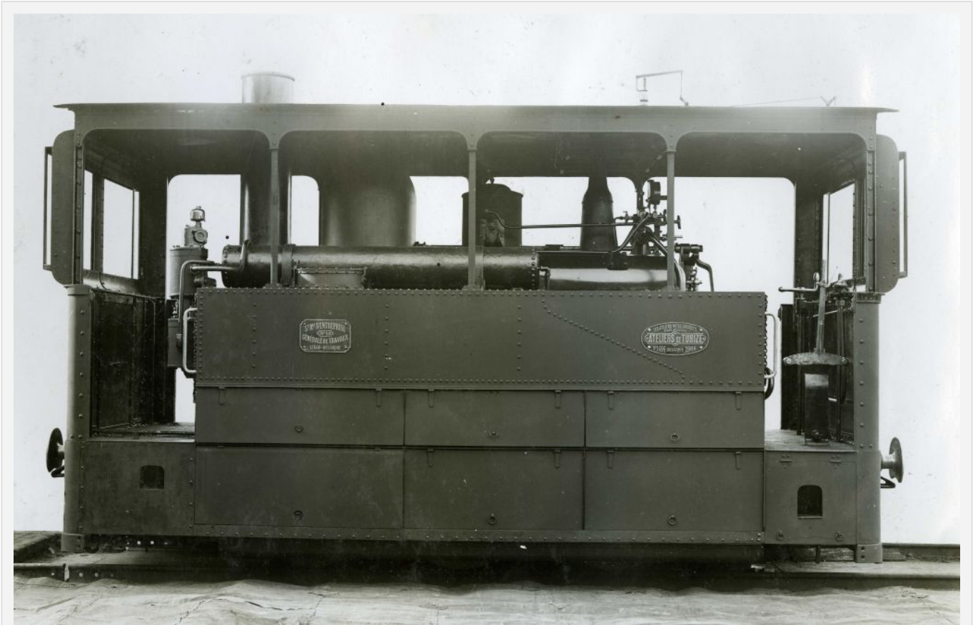
Tubize 1494 de 1906 pour le TBMO (n° 10). Photographie d'usine, coll. Musée 'de la Porte' à Tubize.
