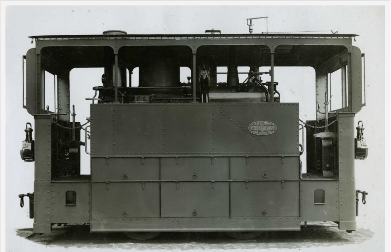
Tubize 1401 de 1904 pour les Tramways à vapeur Vlissinge – Middelburg (n° 5). Photographie d'usine, coll. Musée 'de la Porte' à Tubize.
